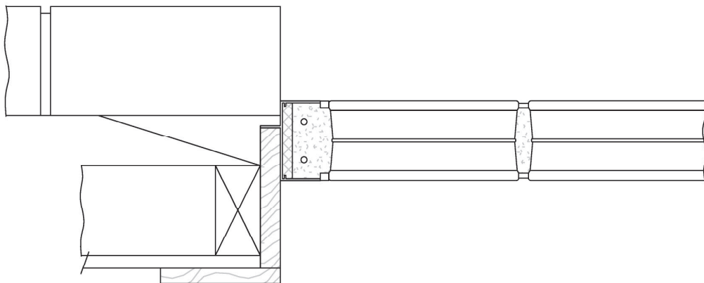
JAMB
